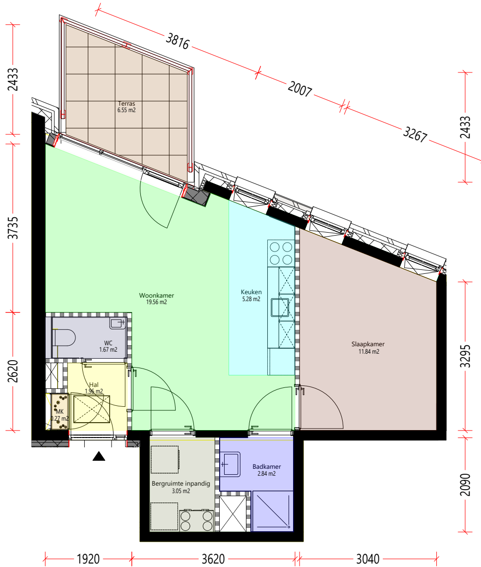
Begane grond
