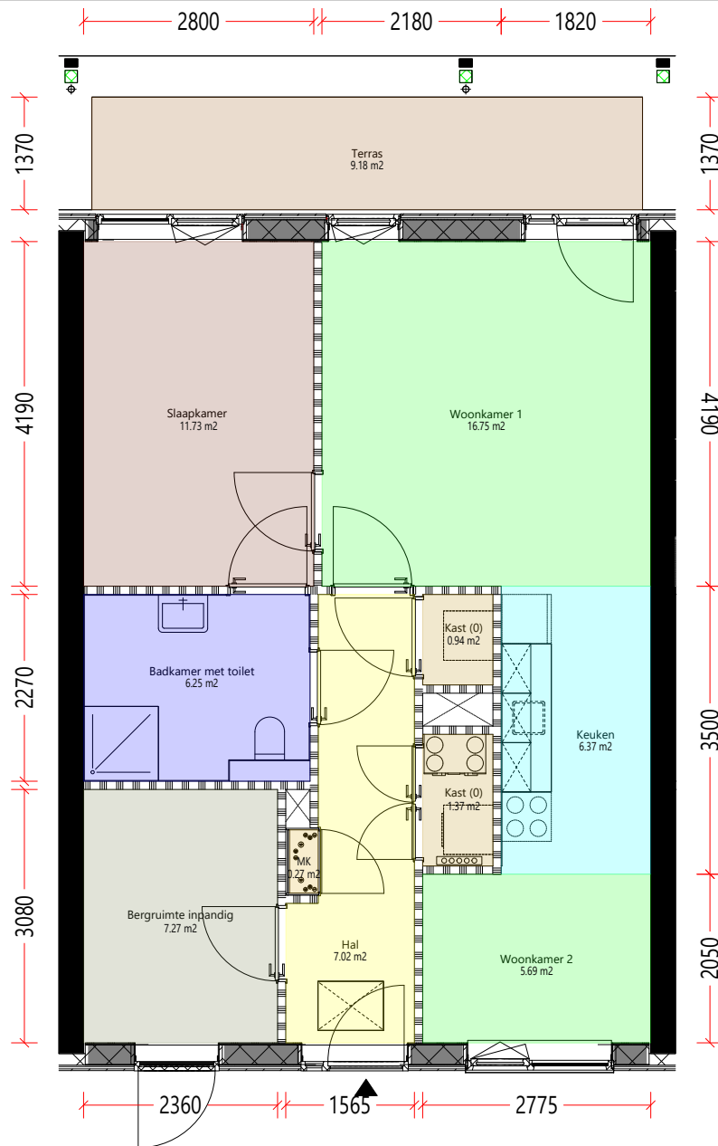
Begane grond
