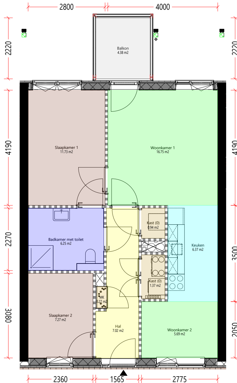
Verdieping_1e
